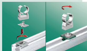
Für BIS RapidStrut®
