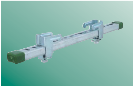
BIS Carril WMO set ligero
