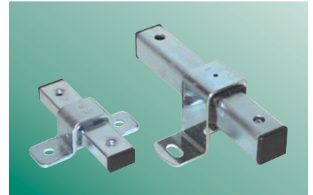
BIS Ekspansionsbeslag U
