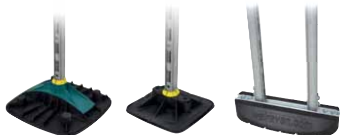
Walraven Yeti® 480
