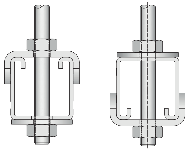
Afbeelding 3: Gebruik van Walraven Strut Onderlegplaat - U-vormig aan de open zijde van de rail
