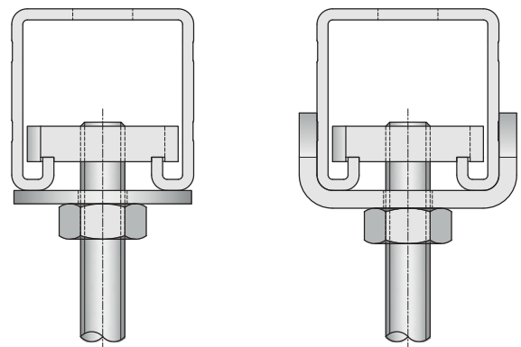
Afbeelding 4: Vergroot de stijfheid van belastingen onder de rail door gebruik te maken van U-vormige onderleggingen (rechter afbeelding) in plaats van standaard platte onderleggingen (linker afbeelding)
