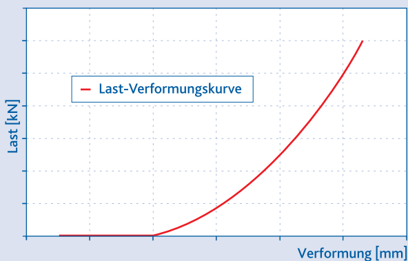
Last-Verformungskurve bis 30 Minuten Brandzeit
