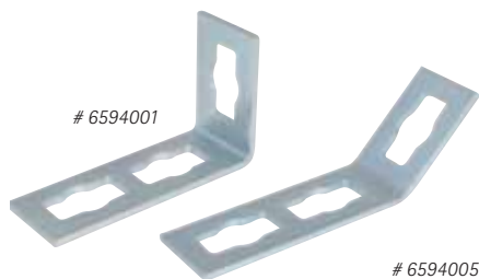
BIS PushStrut Connector Flat 90°/135°
