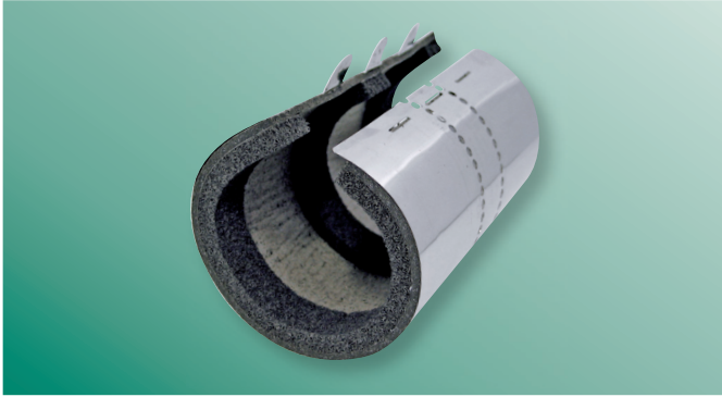
BIS Pacifyre® MK II Brandmanchet Eéndelige inbouwbrandmanchet voor het brandwerend en rookdicht afsluiten van buisdoorvoeringen.
