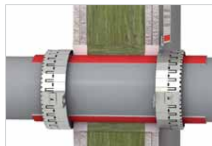
Prostupy sádkovými příčkami s izolací z minerální vlny a použití BIS Pacifyre® FPM protipožární malty.
