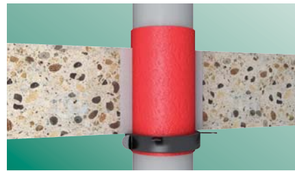
Inbouwsituatie plafonds \geq 150 mm, met PE-isolatie
