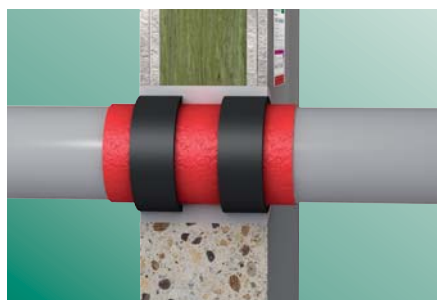
Inbouwsituatie massieve en lichte scheidingswanden \geq 100 mm
