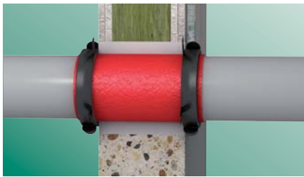
Inbouwsituatie massieve en lichte scheidingswanden \geq 100 mm, met PE-isolatie
