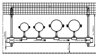
Zavěšená montážní lišta
